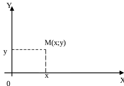
Рис.8.1. Геометрическая интерпретация комплексного числа
