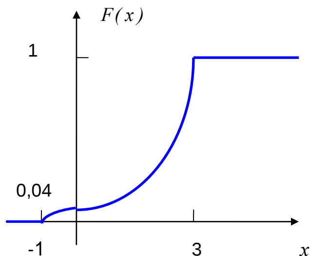
Рис. 3. Функция распределения
